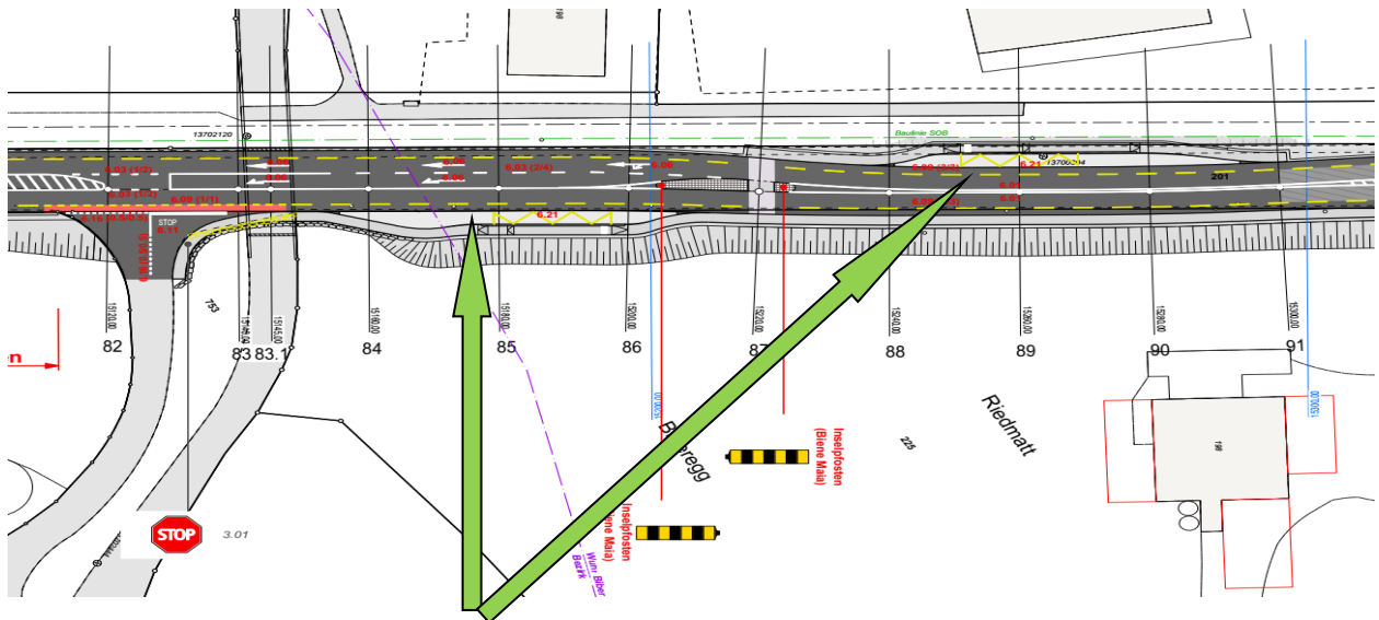
Projektplan der beiden Bushaltestellen mit Strassenüberquerung / Inselposten.
