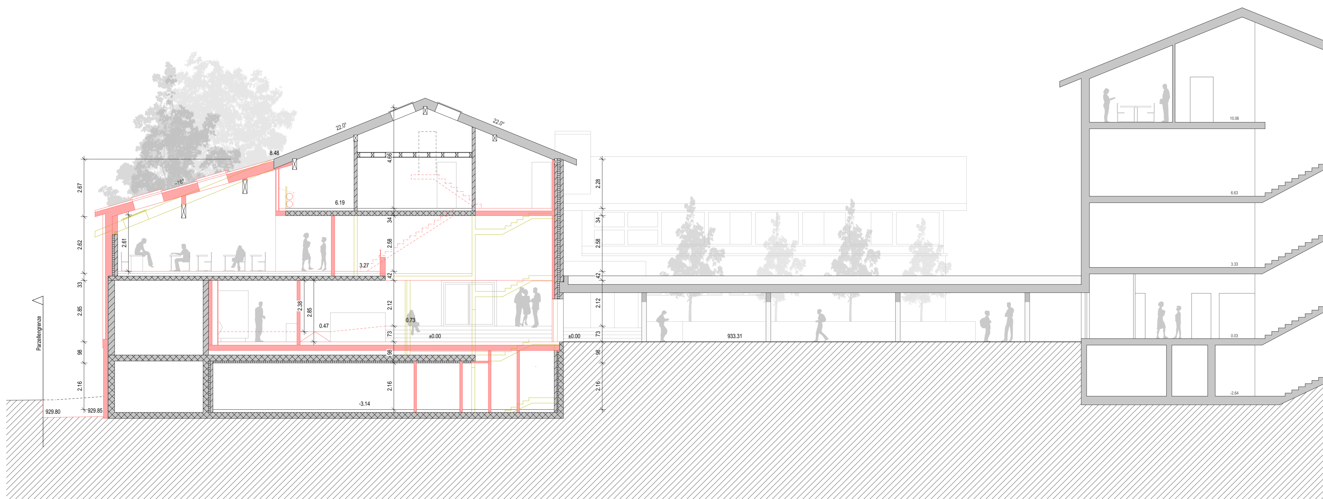
Schnitt B-B
