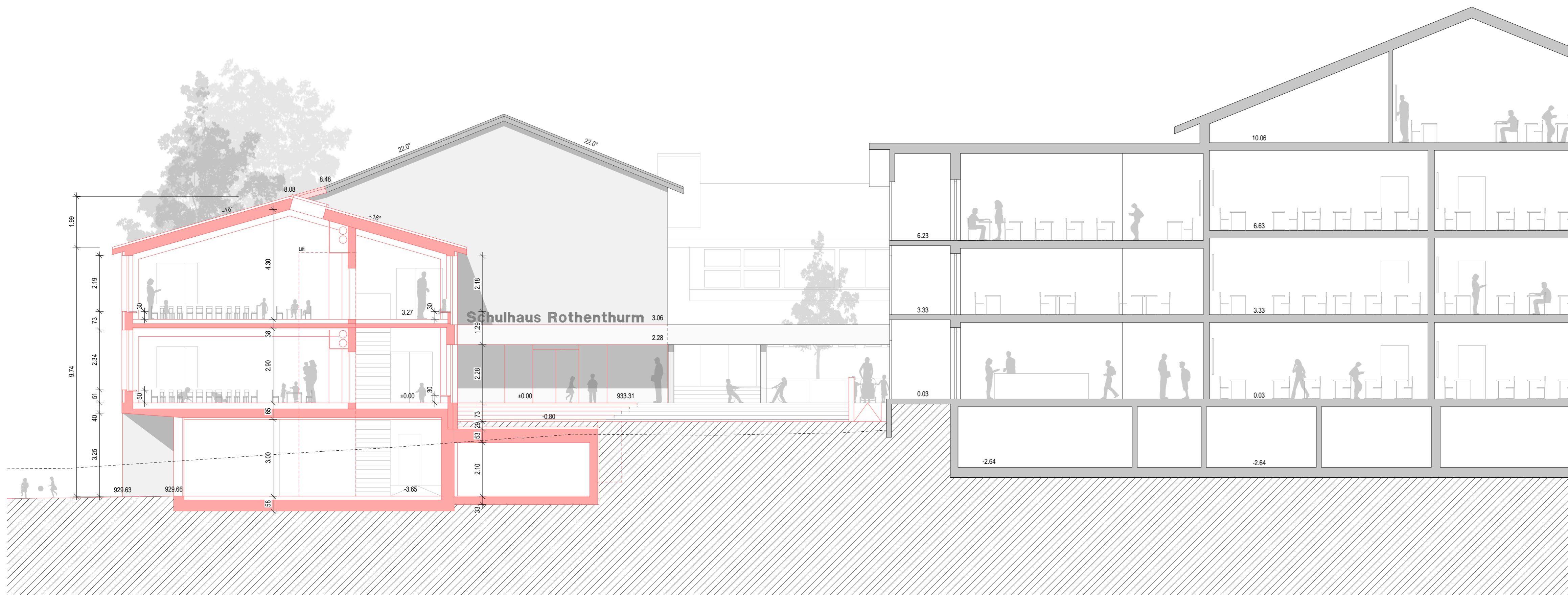
Schnitt A-A
